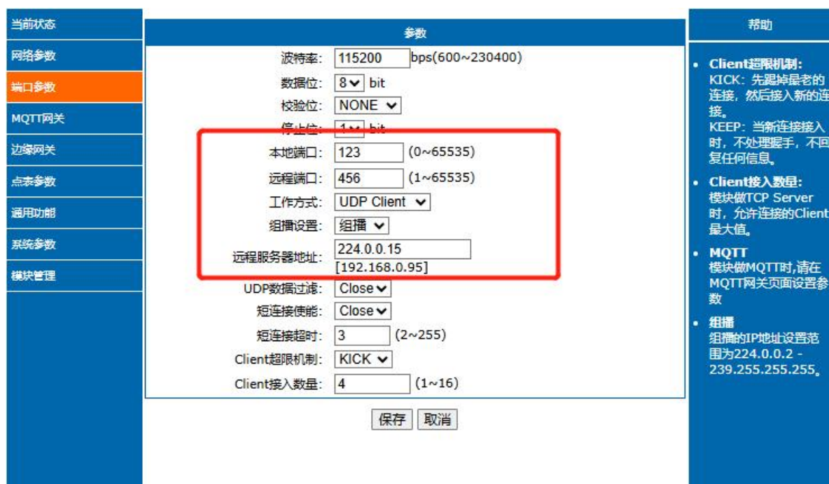
图 24. 组播参数设置
