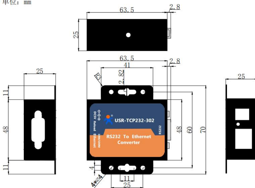
图 1. USR-TCP232-302 尺寸图
