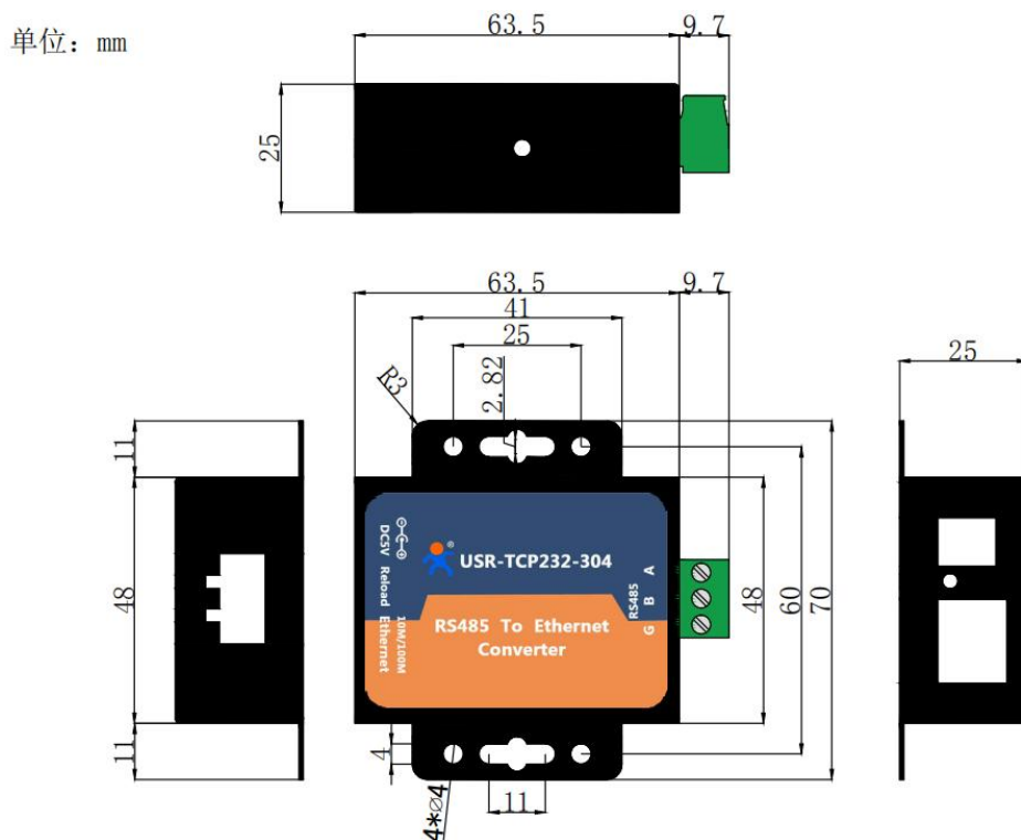
图 2. USR-TCP232-304 尺寸图
