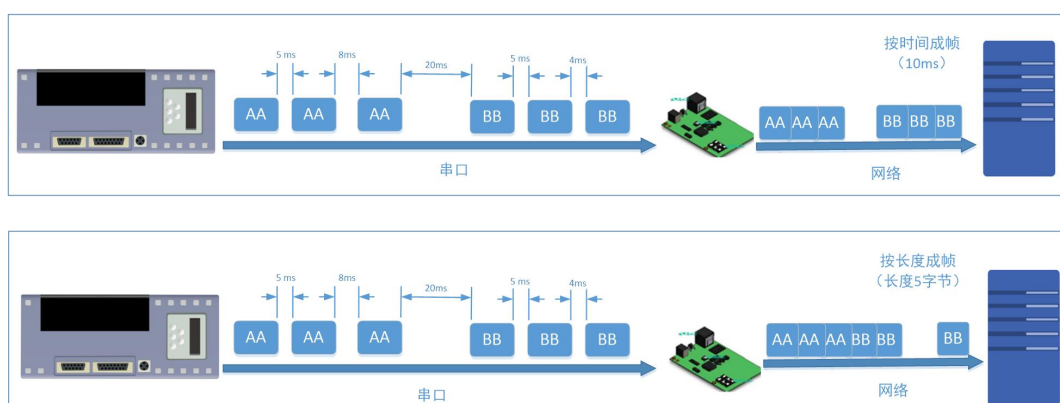
图 8. 端口参数
