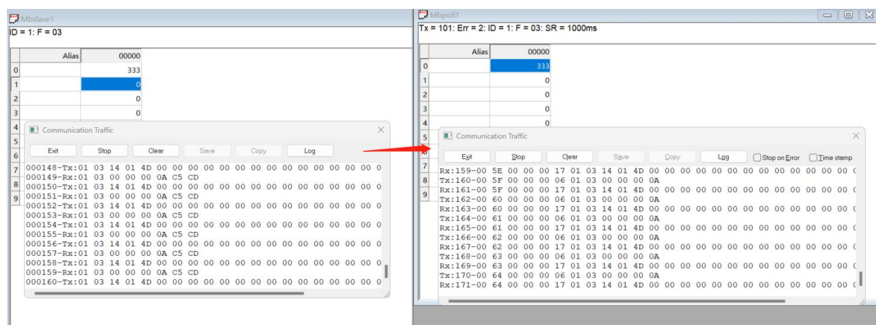
图 45. Modbus RTU 转 Modbus TCP 转换结果
